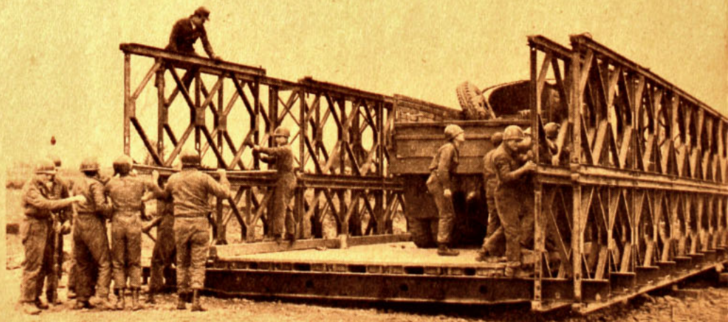
PUENTES AL INSTANTE Ingeniería militar al día.
